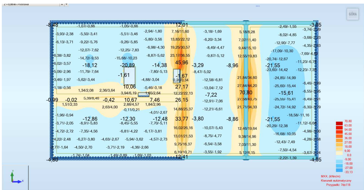
Wyniki momentów zginających Mxx
