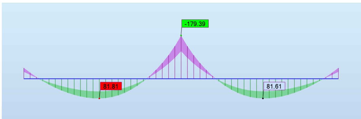
Obwiednia momentów podciągu dwuprzęsłowego
