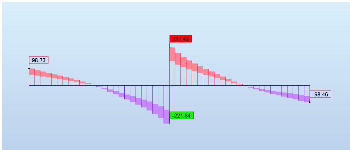
Siły tnące podciągu dwuprzęsłowego
