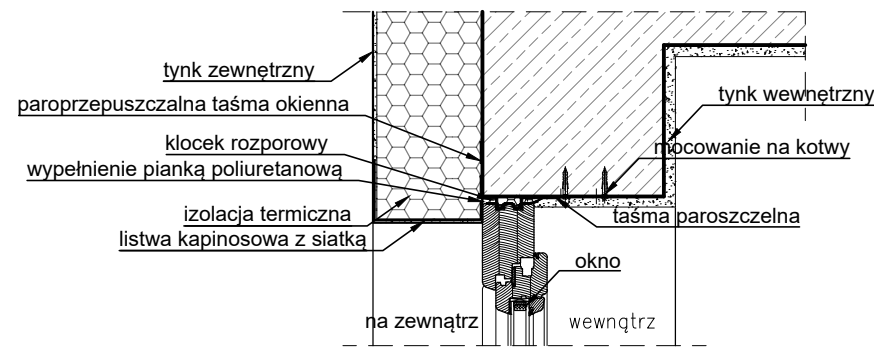
Połączenie okna-ściana-nadproże
