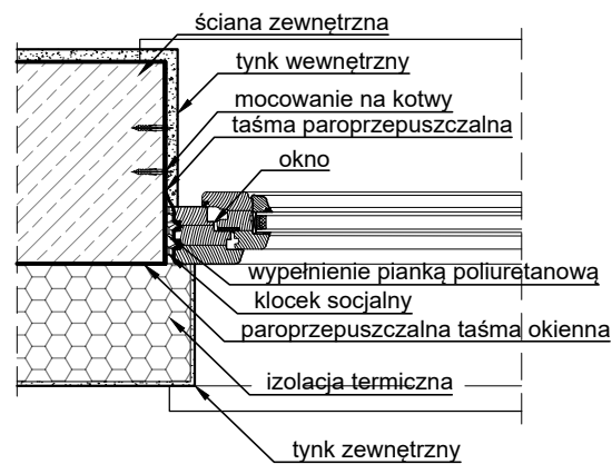
Połączenie okna-ściana
