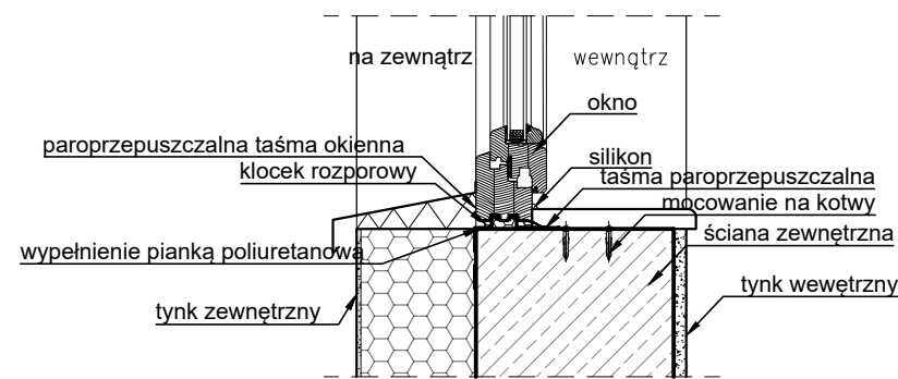
Połączenie okna-ściana-parapet
