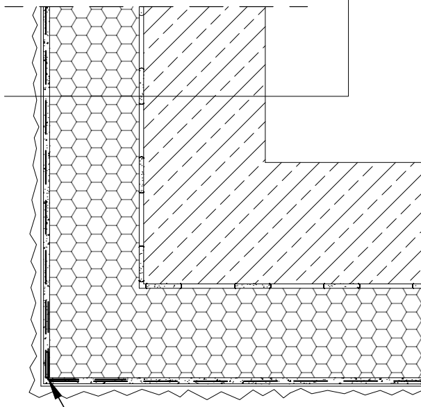
Listwa narożna z siatką 10 x 10 cm
